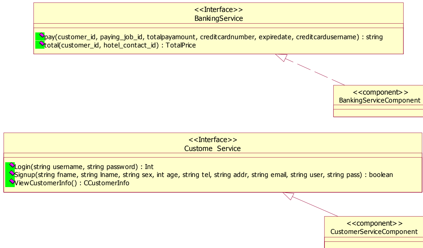
รูปที่ 7-31 Class Diagram ระบบสตูดิโอถ่ายภาพ ส่วนที่1
